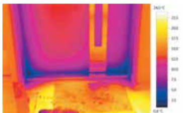
Zdjęcie z kamery termowizyjnej.
